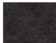
Larvikita
